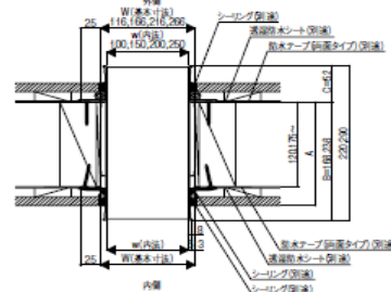
見込み220-290タイプ横断面図
