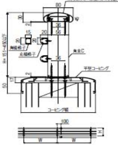
角束C(2段格子)
